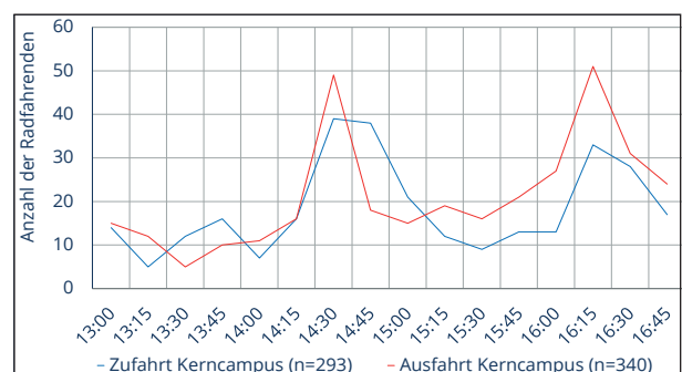
Abb. 73: Ganglinie George-Bähr-Straße / Fritz-Foerster-Platz (eigene Erhebung: videobasierte Verkehrszählung)
