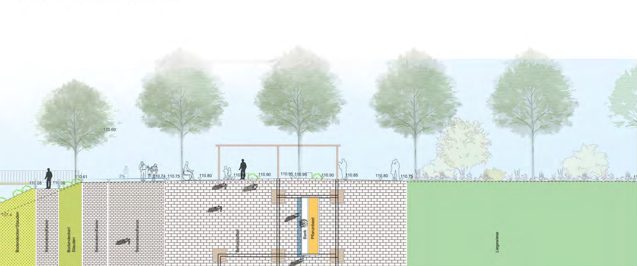
Schnitt Promenade Elbeufer 1:200
