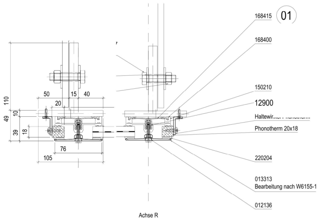
Bild 3.1 Horizontalschnitt Glasaufleger links und rechts
