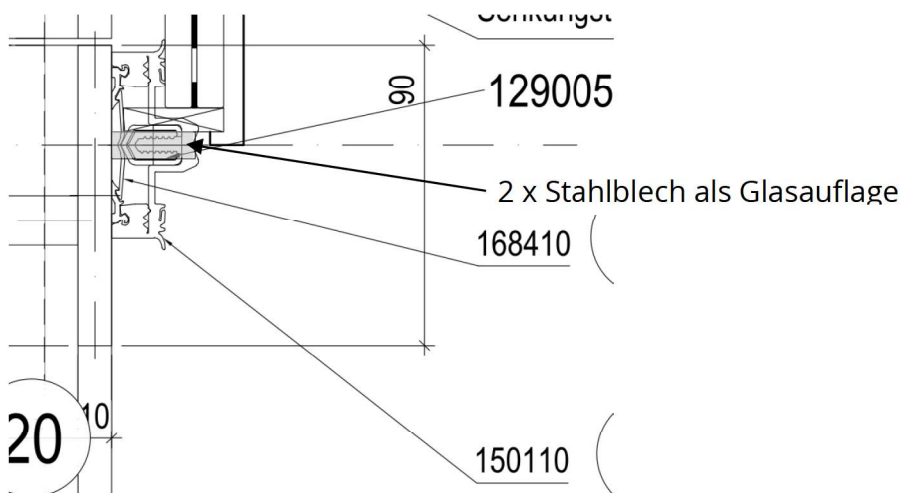
Bild 2 Vertikalschnitt Glasaufleger unten
