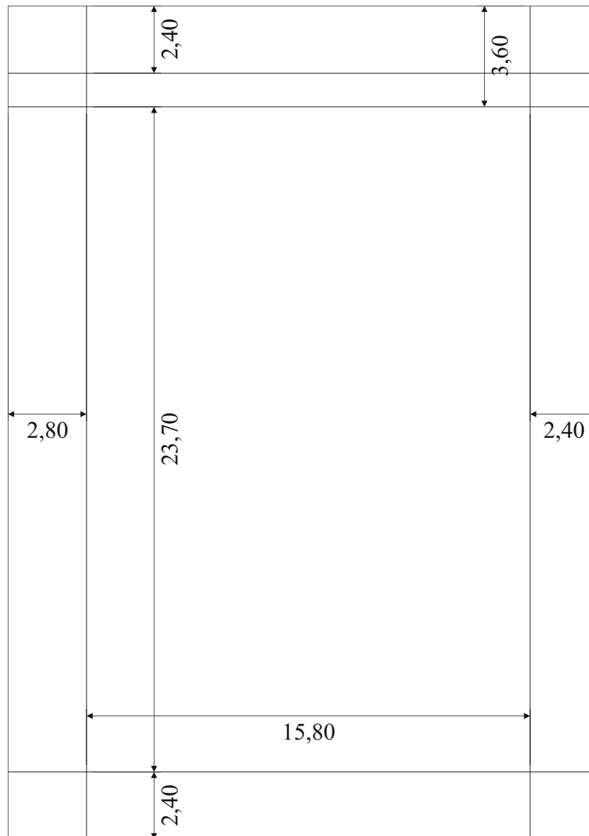
Abbildung A.3: Seitenlayout (Maßangaben in cm)
