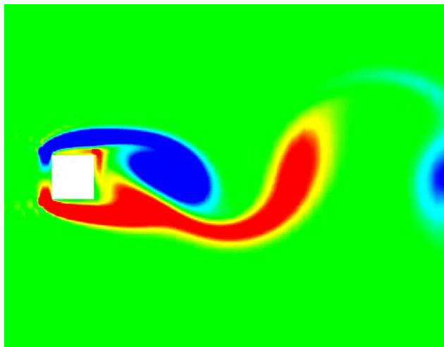
Re = 200
